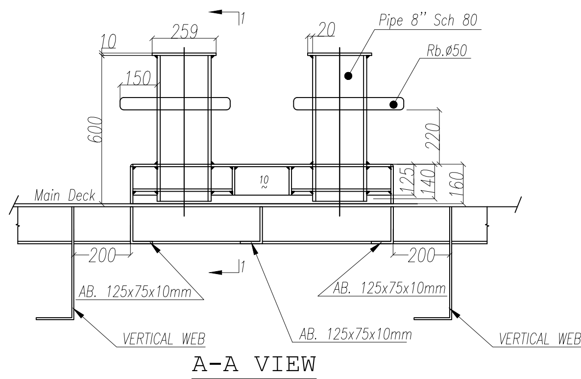
A-A VIEW
